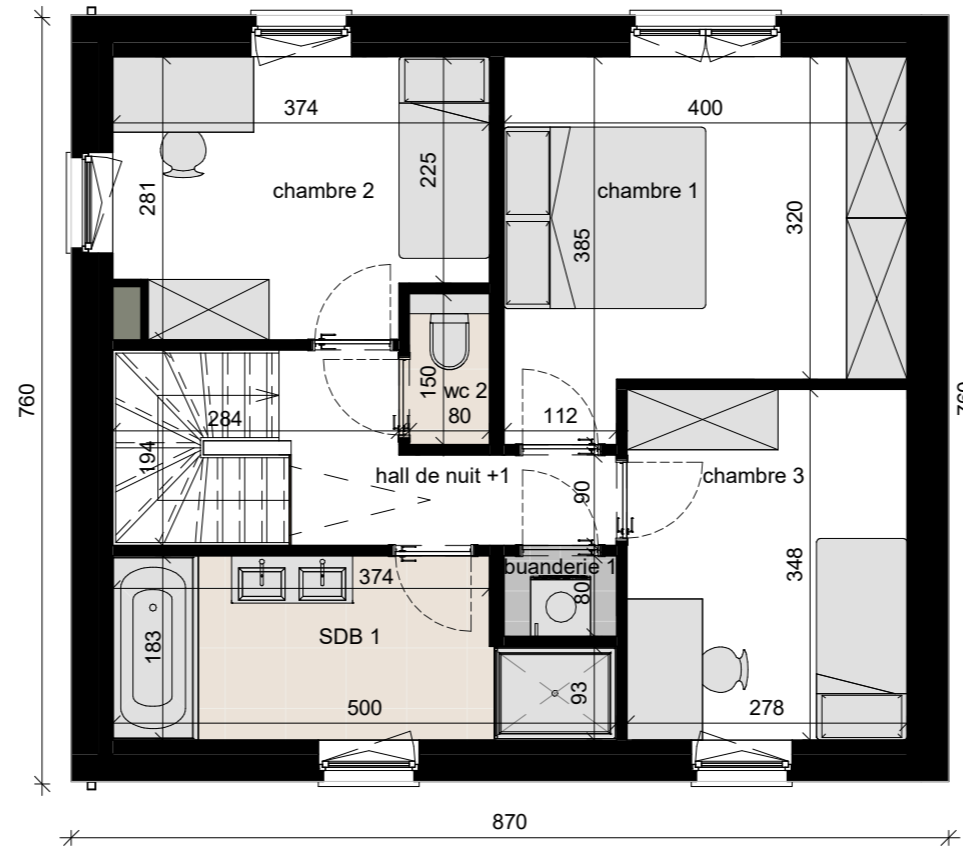
étage surf. brute 66.12 m 2
