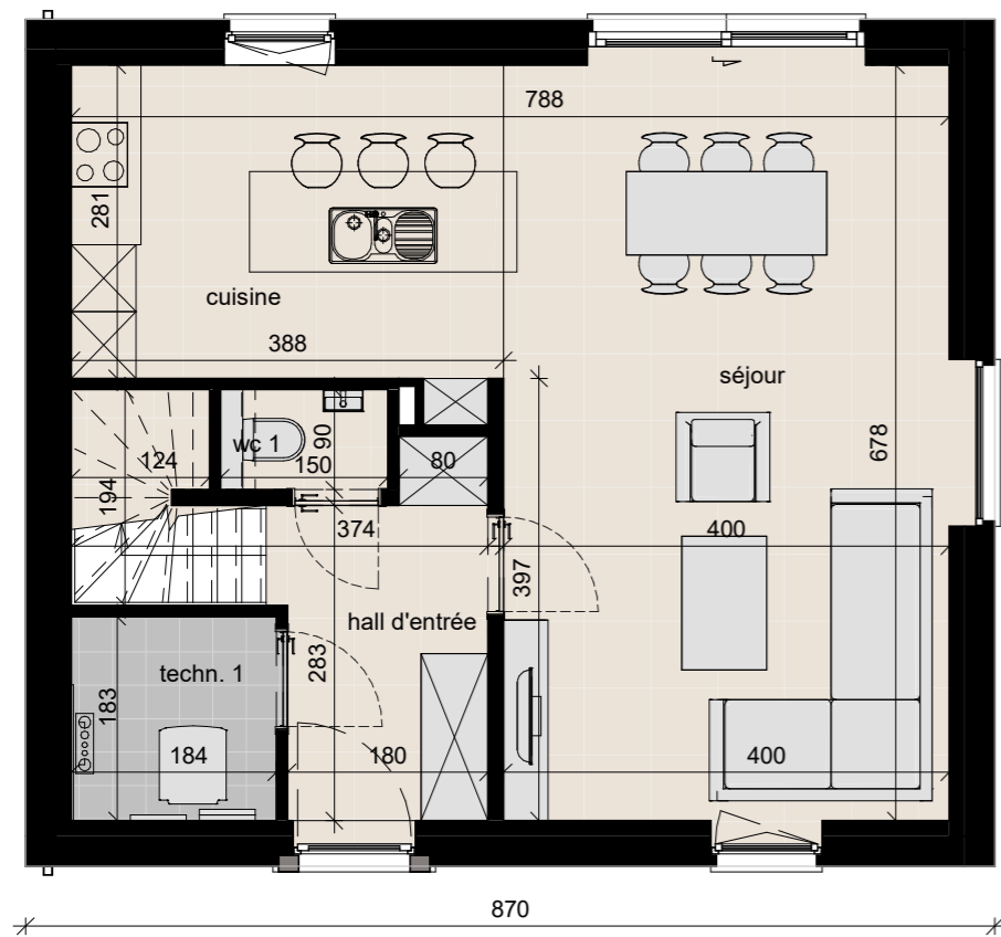
rez-de-chaussée surf. brute 66.12 m 2
